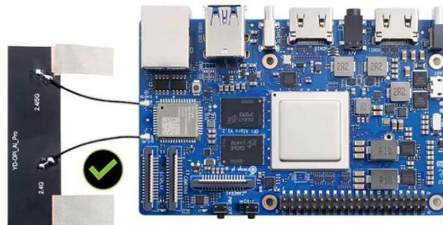
※天线正确安装和使用放置示意图。
